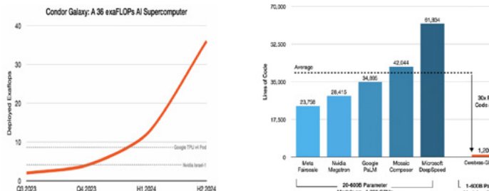
Figura 21. Evolución del Condor Galaxy y su impacto en el entrenamiento de modelos de IA generativa. Fuente: https://www.cerebras.net/blog/introducing-condor-galaxy-1-a-4-exaflop-supercomputer-for-generative-ai/
